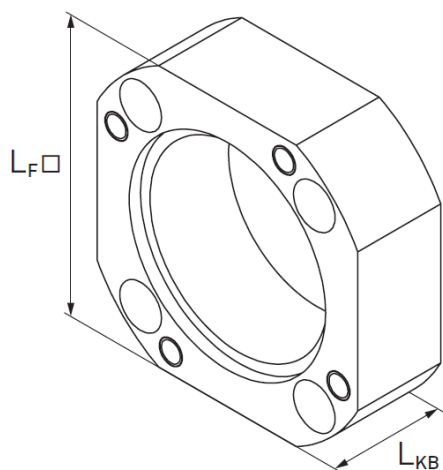
Fig. 11.11 : Carters d'accouplement KB pour modules linéaires HM-B et bras mobile HC-B
