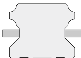
Fig. 4.11 : Éléments de serrage fermé (0 bar)
