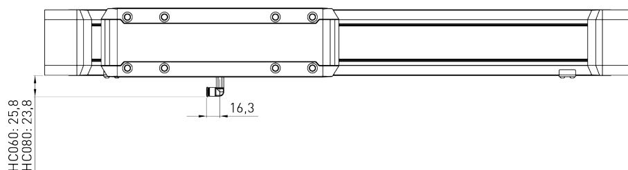
Fig. 6.110 : Position du raccord pneumatique pour l'élément de serrage ou de freinage (HC060B, HC080B)
