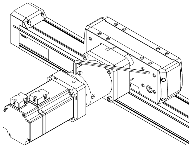
Fig. 6.98 : Serrage du moyeu de serrage sur l'arbre du moteur
