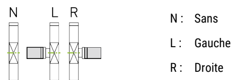
Fig. 4.17 : Interfaces d'entraînement de l'axe linéaire HC-B
