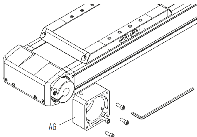
Fig. 6.77 : Montage de la plaque d'adaptation du réducteur AG – HT150B, HT200B, HT250B
