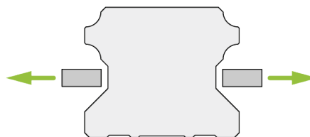
Fig. 4.14 : Éléments de freinage ouvert (5,5 à 6,5 bar)
