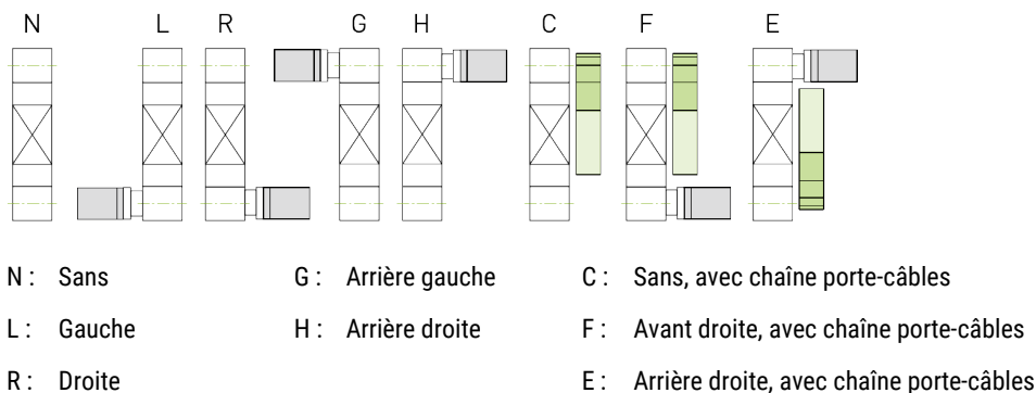
Fig. 4.16 : Interface d'entraînement de l'axe linéaire HT-B
