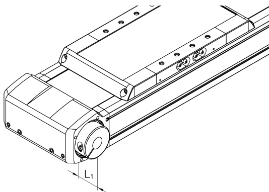
Fig. 6.71 : Réglage distance moyeu de serrage direction moteur
