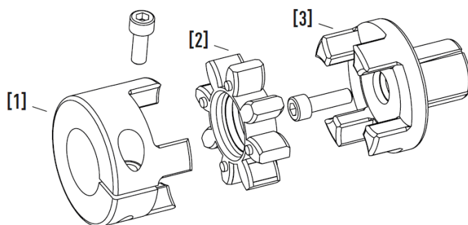
Fig. 6.67 : Variante 2 du bloc d'accouplement : Moyeu de serrage avec deux vis de serrage
