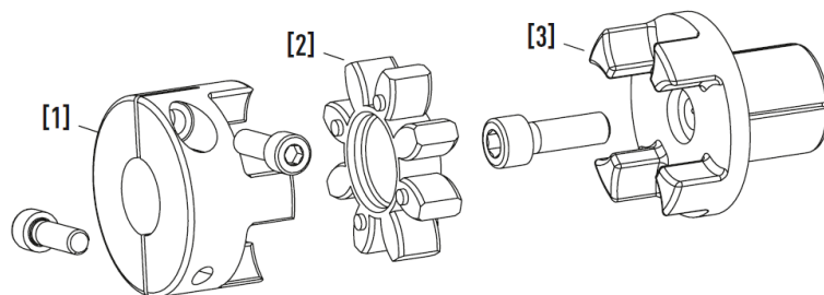
Fig. 6.67 : Variante 2 du bloc d'accouplement : Moyeu de serrage avec deux vis de serrage
