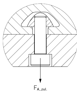
Fig. 6.22 : Fixation avec coulisseaux – HT100B, HT150B
