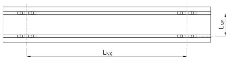
Fig. 6.22 : Fixation avec coulisseaux – HT100B, HT150B
