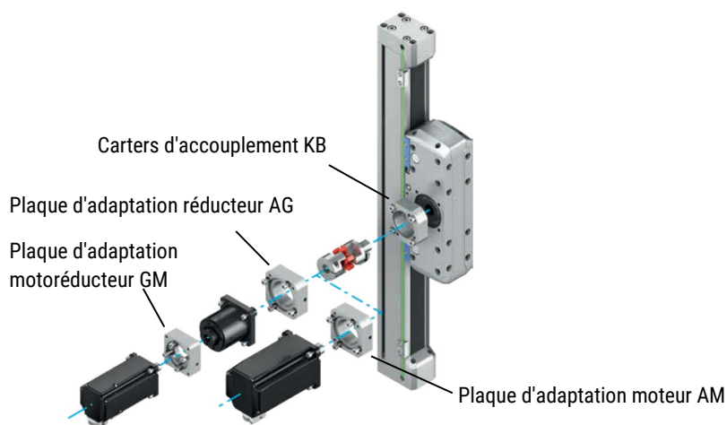
Fig. 11.4 : Adaptateur moteur du bras mobile HC
