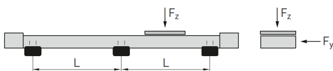
Fig. 6.7 : Position de l'axe à l'horizontale
