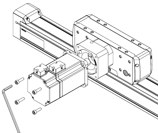
Fig. 6.91 : Vissage du moteur sur l'axe cantilever HC-B
