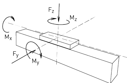
Fig. 7.3 : Illustration des forces et des couples sur l'axe portique à chariot fixe
