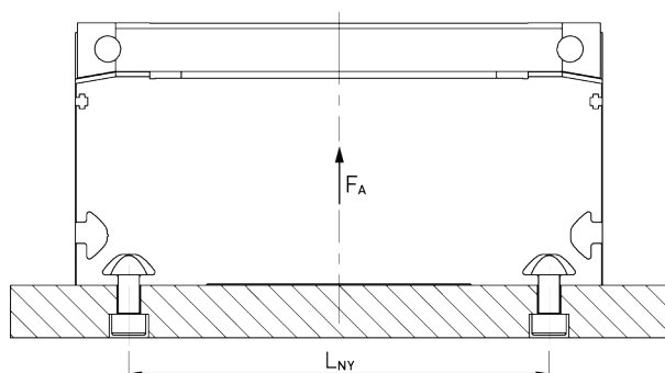
Fig. 6.19 : Espacement des trous pour la fixation des tables linéaires HT100B, HT150B, HT200B par le bas avec des coulisseaux
