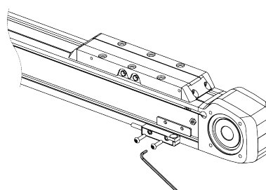
Fig. 6.39 : Montage du capteur fin de course : HM040, HT100
